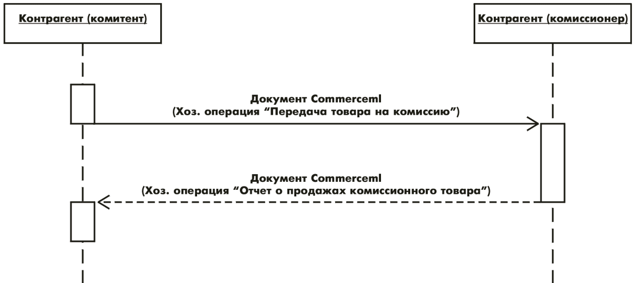
Рис.7 Схема обмена документами Commercetl при передаче товара на комиссию и отчетах комиссионера
